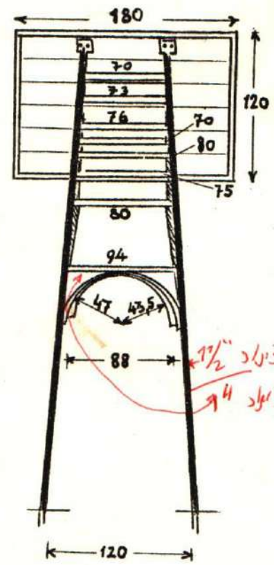
המבנה התומך בלוח הסל בקו מאוזן
