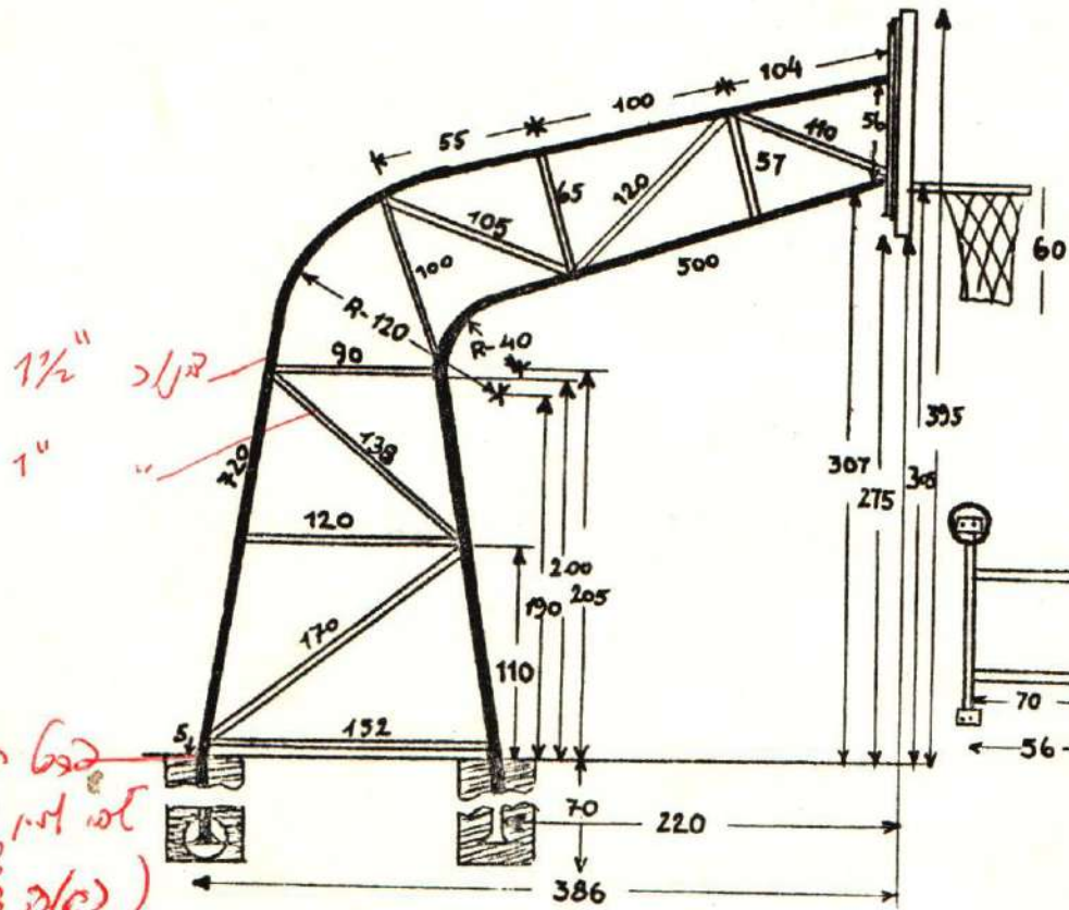
מבנה הקונסטרוקציה הסומכת את לוח הסל
