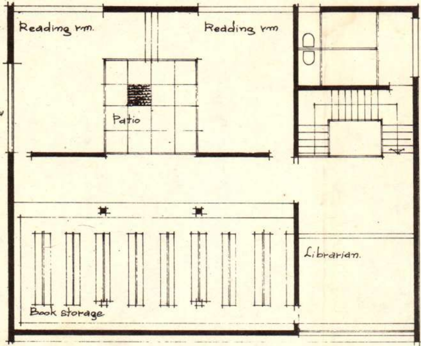
Upper floor plan 1:100 תכנית ק"ג
