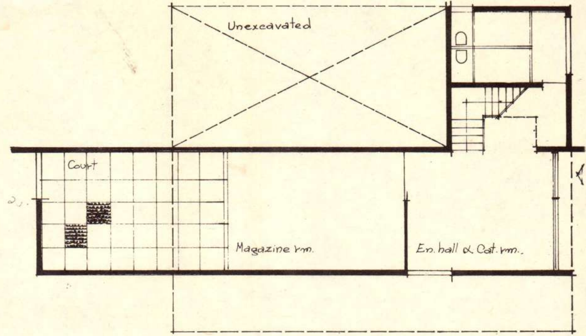
Ground floor plan 1:100 תכנית ק קרקע
