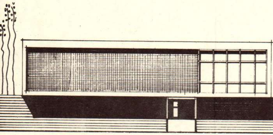
Eastern elevation 1:100 חזית מזרחית
